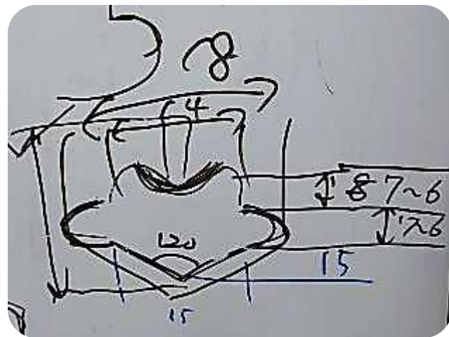
コマの設計
